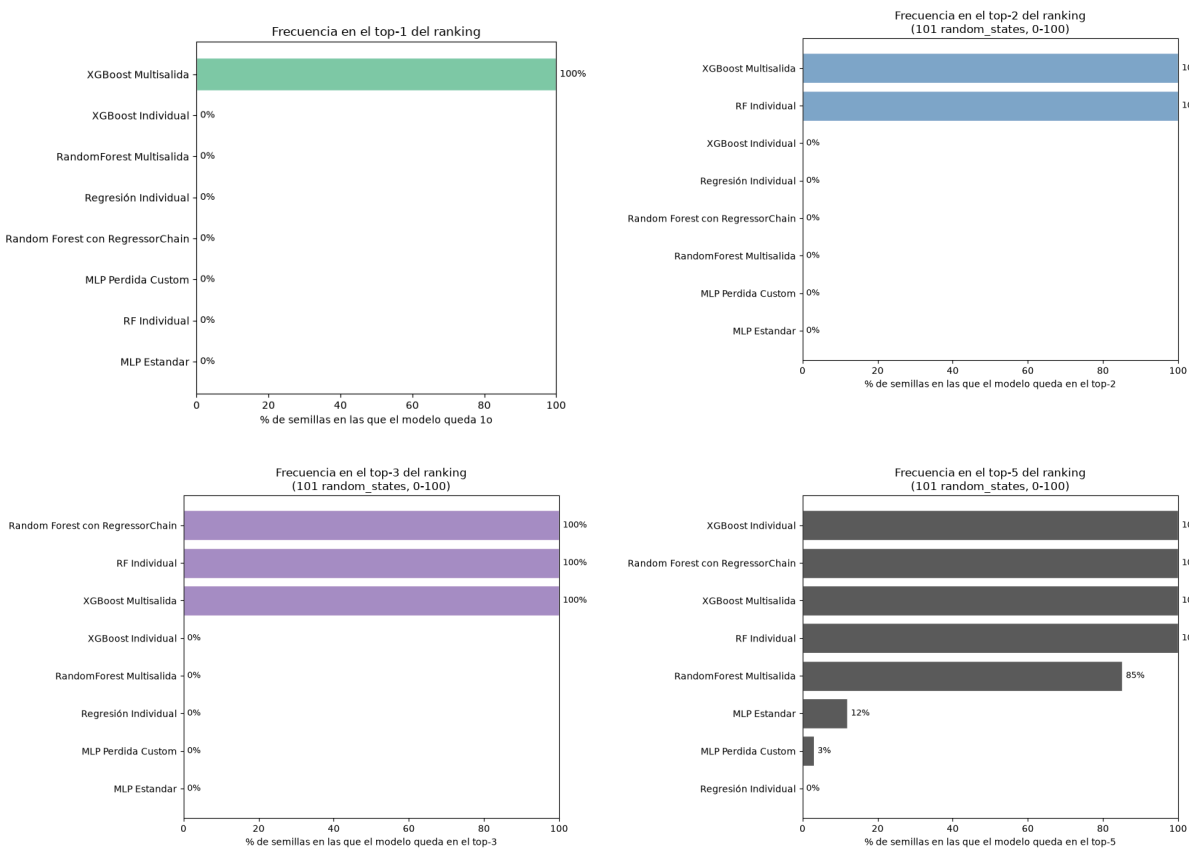
Figura 8: Gráficas de top 1, 2, 3 y 5 en base al porcentaje de veces que un modelos se encuentra dentro de ese top.
