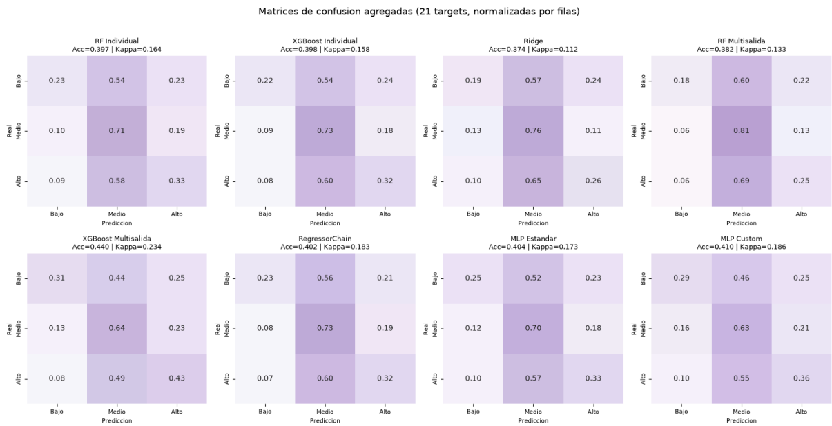
Figura 6: Matrices de confusión.
